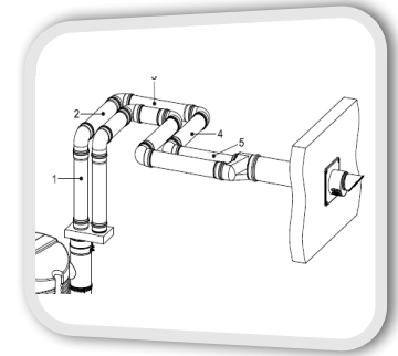
Įvairios kamino įrengimo galimybės
