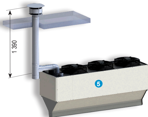
Kaminas per stogą B22
