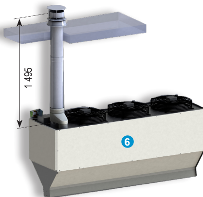
Koncentrinis kaminas per stogą C32
