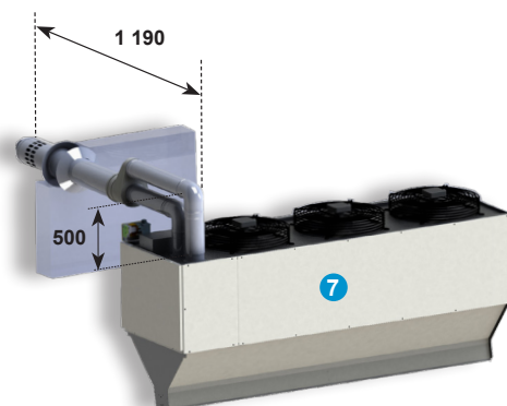
Koncentrinis kaminas per sieną C12
