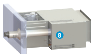
Koncentrinis kaminas per sieną C12 maksimalus ilgis : 6m
