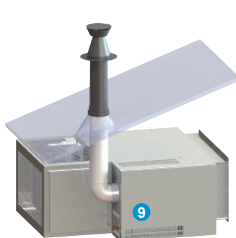
Koncentrinis kaminas per stogą C32 maksimalus ilgis : 6m
