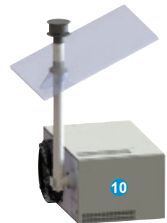
Kaminas per stogą B22 maksimalus ilgis : 8m
