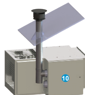
Kaminas per stogą B22 maksimalus ilgis : 8m
