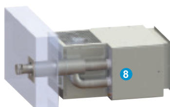
Koncentrinis kaminas per sieną C12 maksimalus ilgis : 6m
