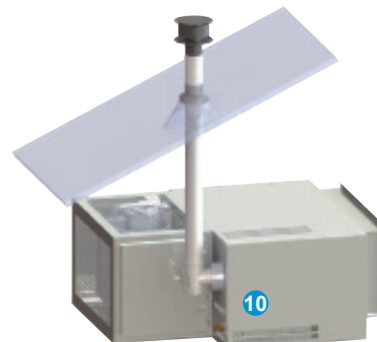
Kaminas per stogą B22 maksimalus ilgis : 8m
