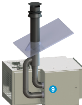
Koncentrinis kaminas per stogą C32 maksimalus ilgis : 8m
