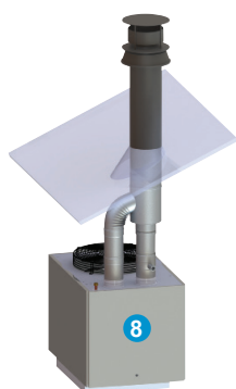
Koncentrinis kaminas per stogą C32 maksimalus ilgis : 8m
